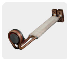
Fokussierungsspule rund frontal (Bestell-Nr.09-119-01)
